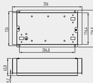
Szeregowo-równoległy moduł wej./wyj. do jednostki wewnętrznej (CZ-CAPBC2)
