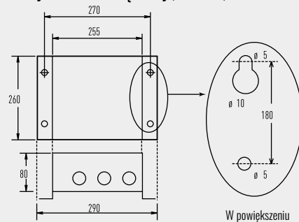
Szeregowo-równoległy moduł wej./wyj. do jednostki zewnętrznej (CZ-CAPDC2)
