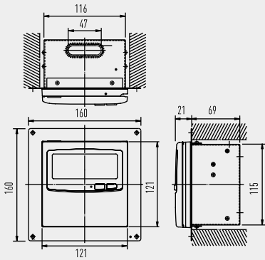
Sterownik systemowy (CZ-64ESMC2)
