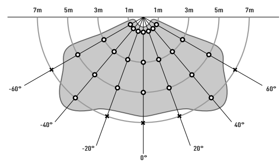
Obszar detekcji osób (wysokość 2,5 m, kąt 30^{\circ} )
